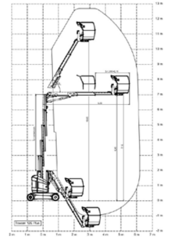
Werkbereik 12,7 m
