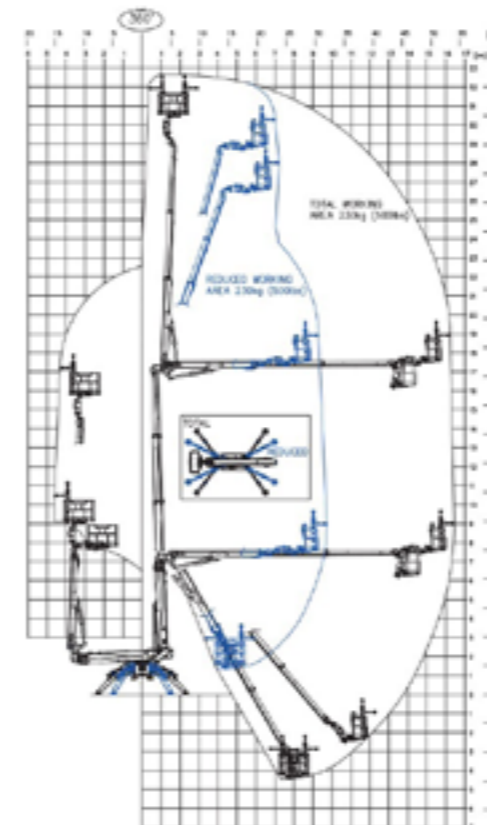
Werkbereik 33 m
