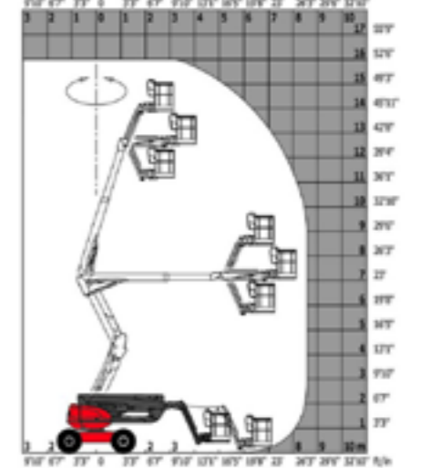
Werkbereik 20 m
