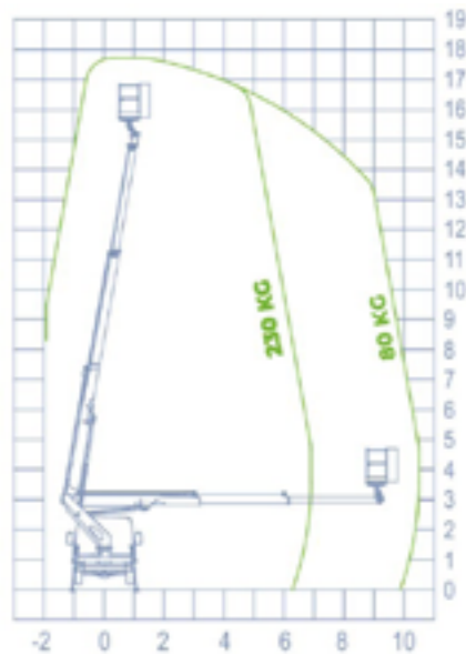
Werkbereik 18 m
