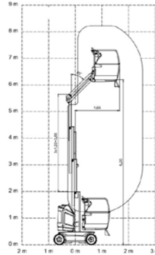
Werkbereik 8 m
