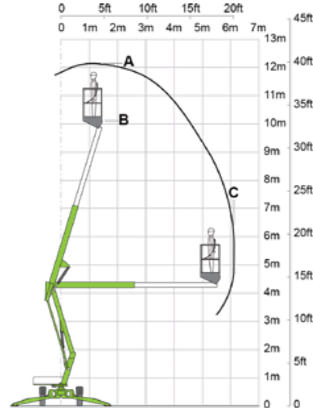
Werkbereik 12,3 m
