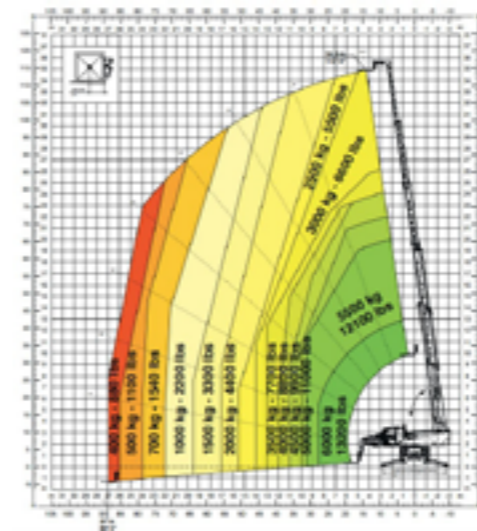
Werkbereik 8T 46 m
