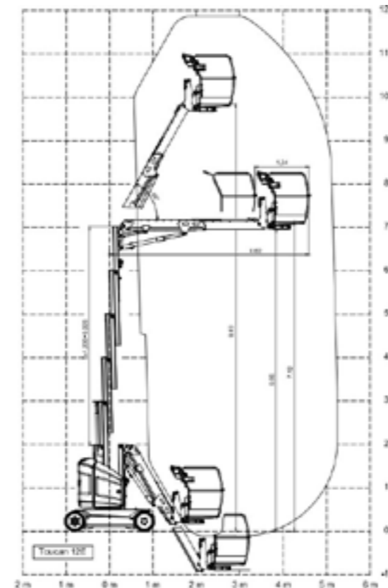
Werkbereik 12 m
