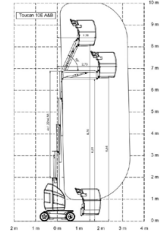
Werkbereik 10 m
