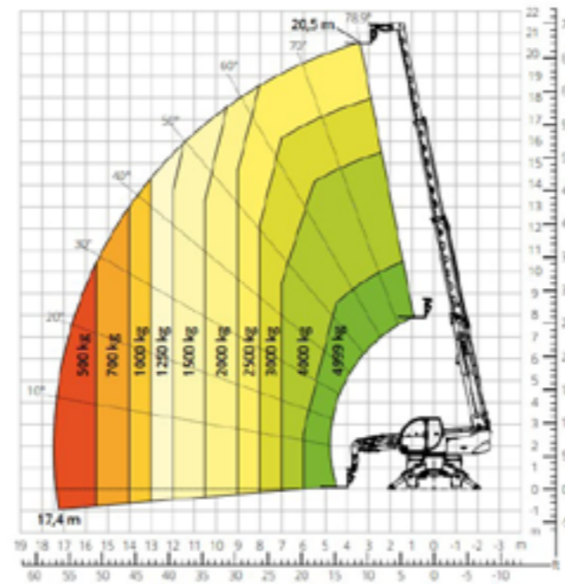
Werkbereik 5T 21 m
