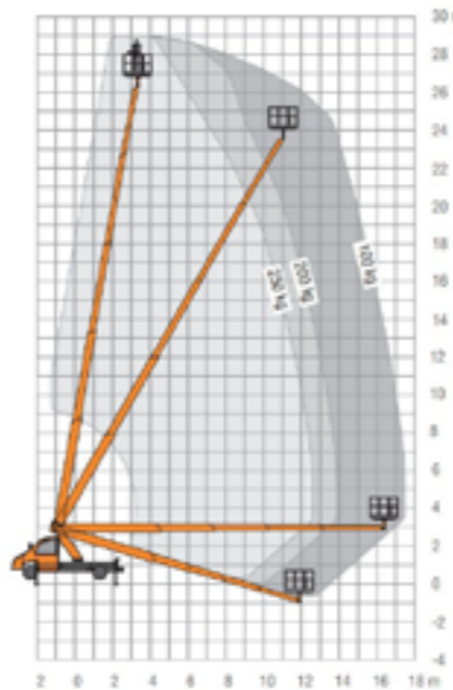
Werkbereik 29 m
