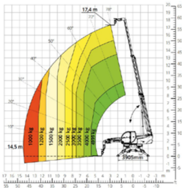
Werkbereik 4T 18 m
