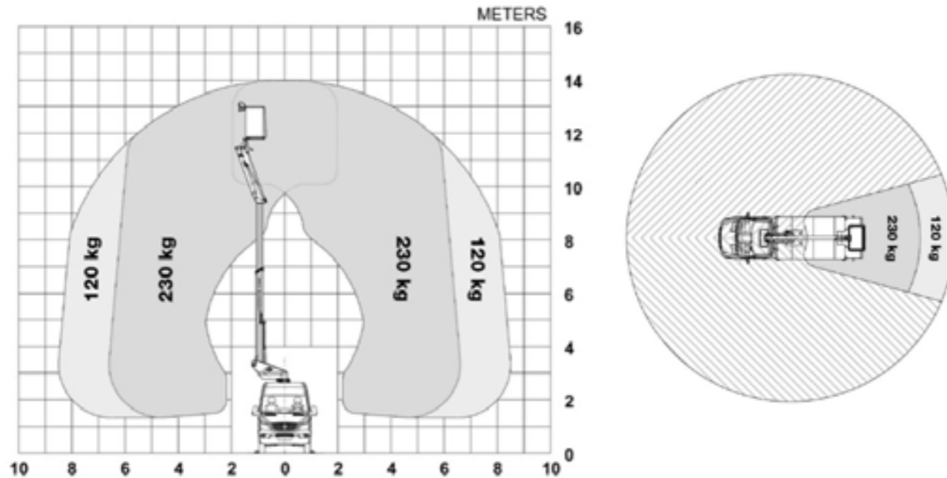
Werkbereik 14,4 m
