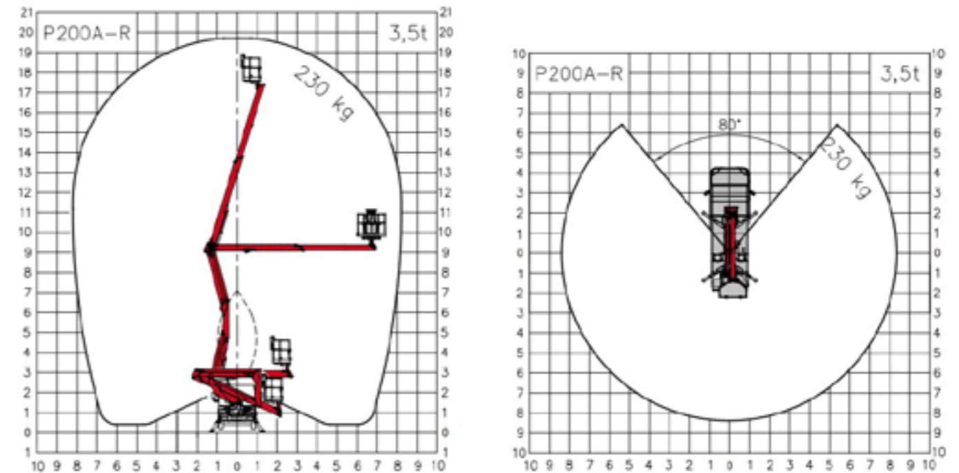
Werkbereik 20 m
