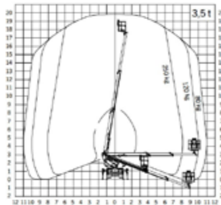
Werkbereik 20 m
