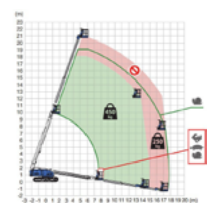
Werkbereik 23 m
