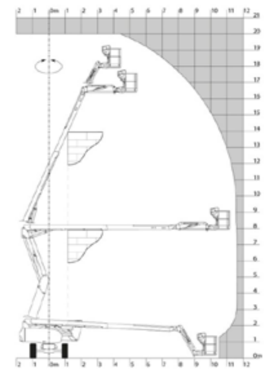
Werkbereik 20 m
