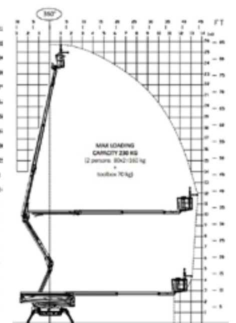
Werkbereik 26 m
