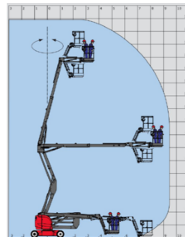
Werkbereik 17 m
