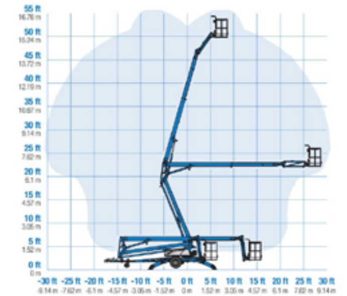
Werkbereik 17 m
