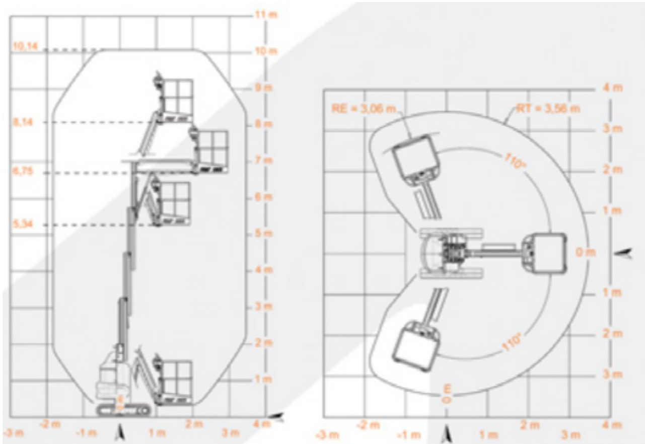
Werkbereik 10 m
