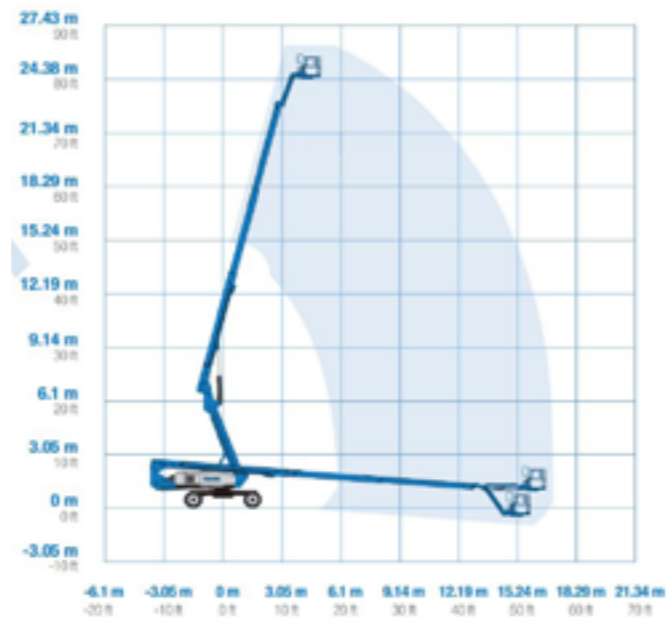
Werkbereik 26,4 m kniktelescoop
