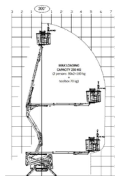
Werkbereik 15 m
