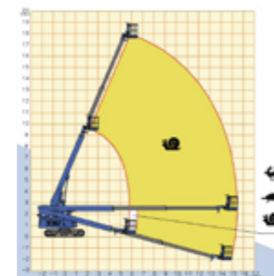
Werkbereik 20 m
