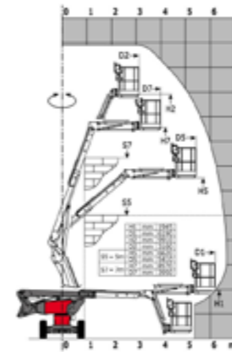
Werkbereik 18 m
