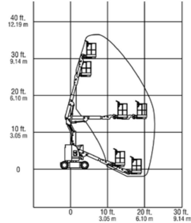
Werkbereik 11 m
