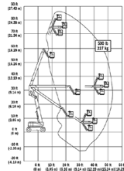
Werkbereik 26 m
