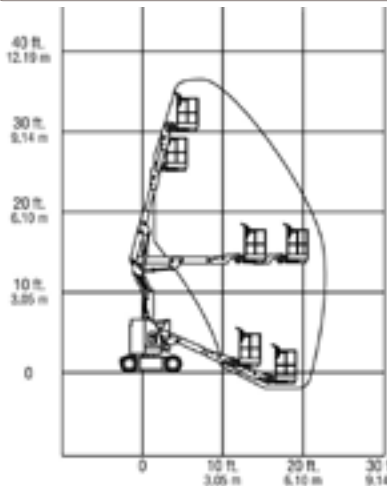
werkbereik 11 m
