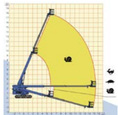
werkbereik 20 m
