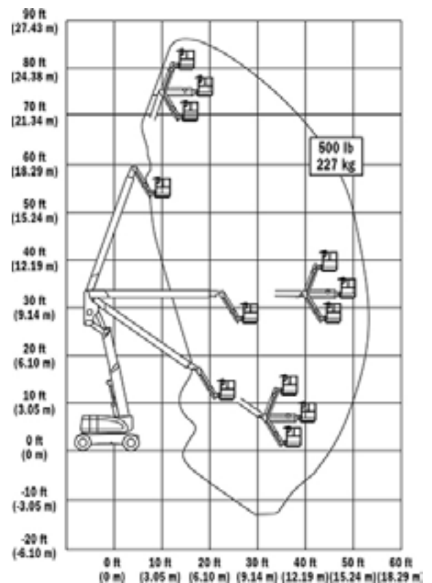
werkbereik 26 m
