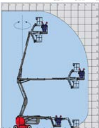
werkbereik 17 m
