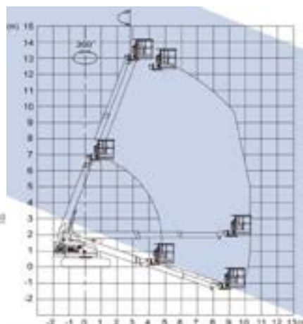
werkbereik 15 m
