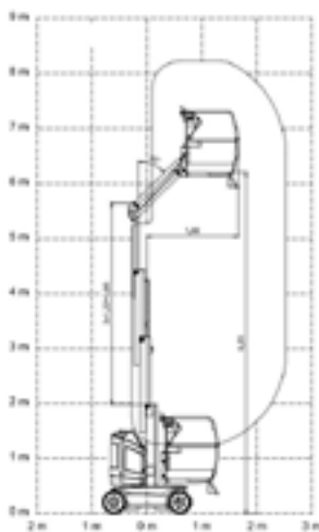
werkbereik 8 m
