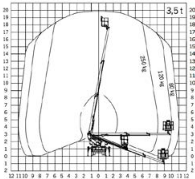
werkbereik 20 m
