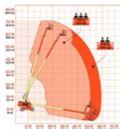
werkbereik 22 m
