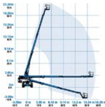
werkbereik 22 m
