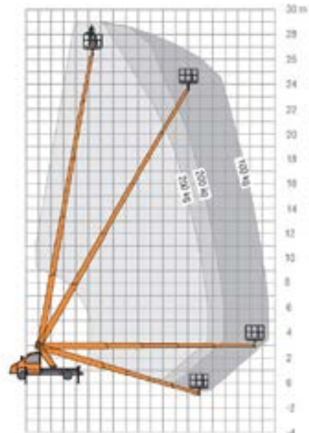
werkbereik 29 m
