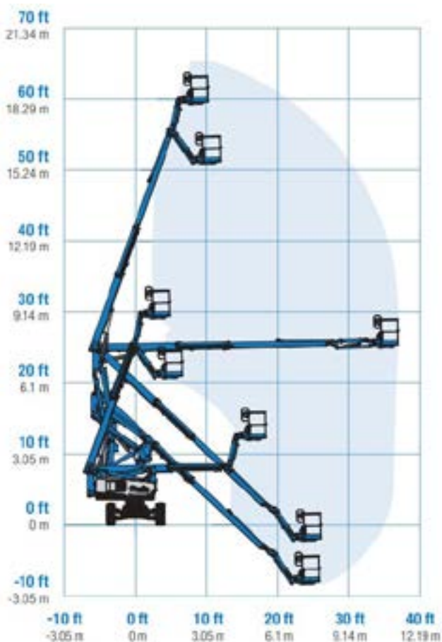
werkbereik 20 m
