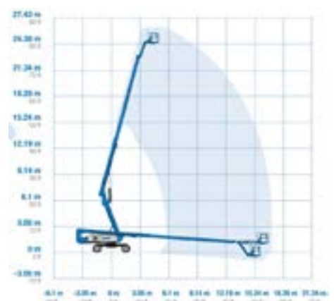
werkbereik 26,4 m kniktelescoop
