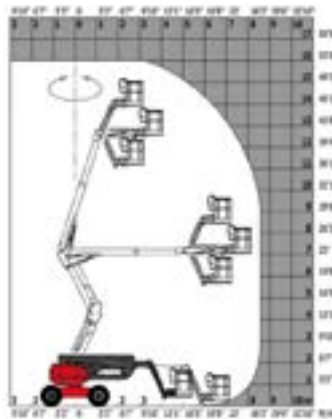
werkbereik 26 m
