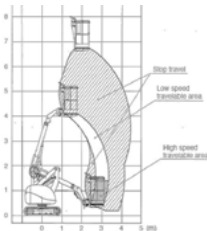
werkbereik 9 m
