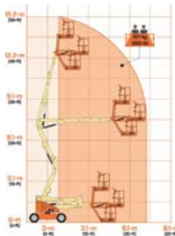
werkbereik 15,5 m
